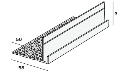
Ventilatie inhaakstartprofiel nr. 2866
