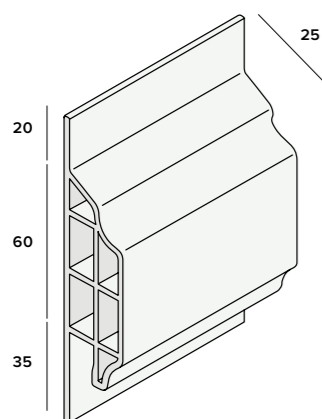
Trim/kraal sierlijst klassiek nr. 2850
