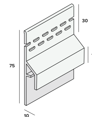
Trim ventilatie dakrand nr. 2833
