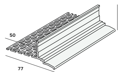
Ventilatie startprofiel nr. 2826
