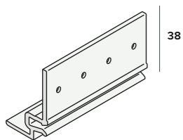
Montageprofiel boeiboord nr. 2887
