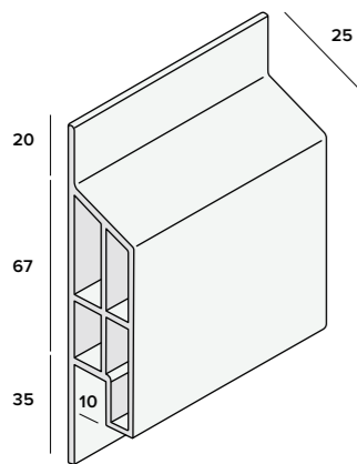
Trim/kraal sierlijst modern nr. 2851
