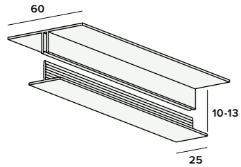
Verbindingprofiel 2-delig nr. 0512
