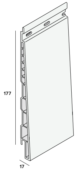
Potdeksel 177 mm nr. 2817
