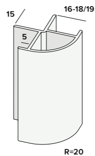
Hoekverbinding 16 mm nr. 0316
