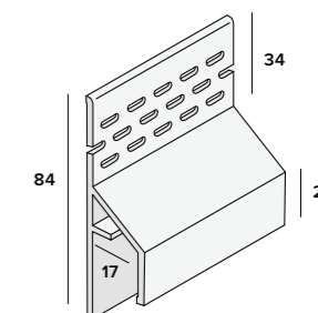
Ventilatie trim/kraalprofiel nr. 2849
