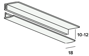
Startprofiel 2-delig nr. 0510
