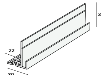
Ventilatie inhaakstartprofiel nr. 2864
